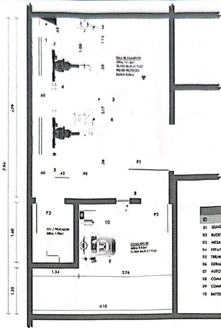
02 PLANTA BAIXA - LAYOUT DE INSTALAÇÃO ESCALA: 1/50
