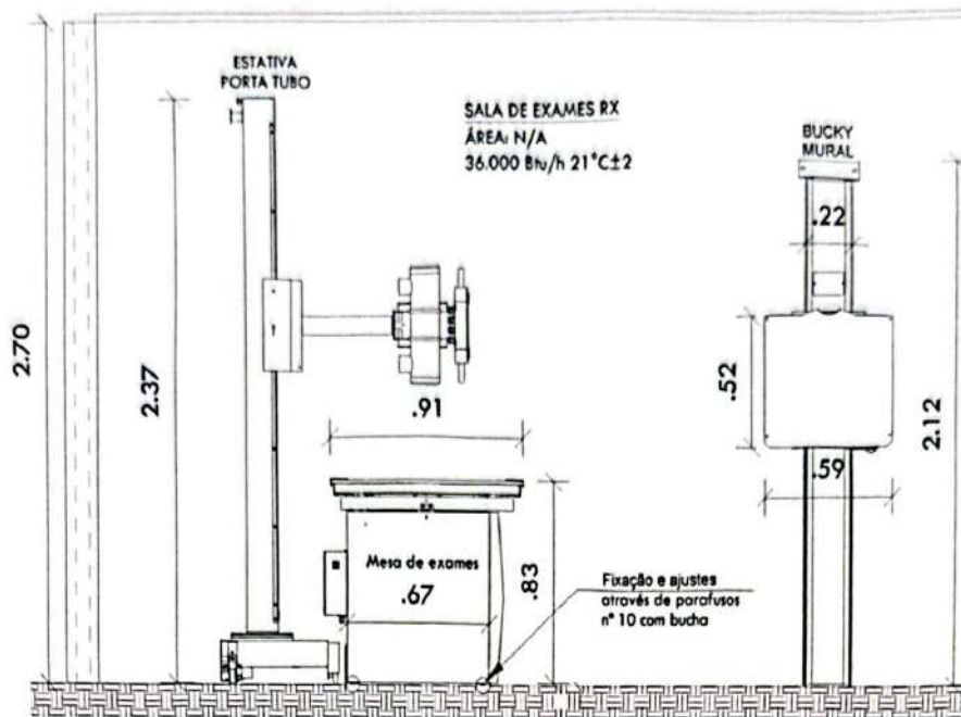
02 VISTA LATERAL DO RAO-X ESCALA: N/A
