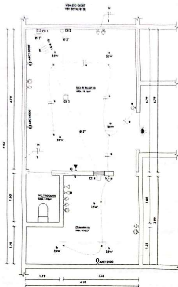
04 PLANTA BAIXA - DETALHES ELÉTRICOS ESCALA: 1/50
